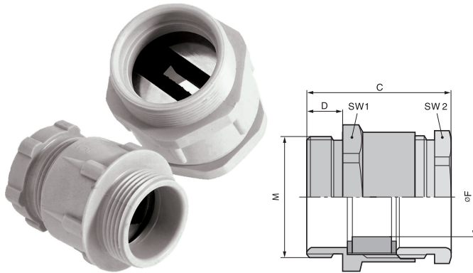
SKINDICHT® SVFK-M
